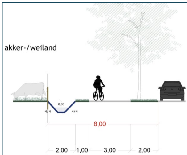
Dwarsprofiel 10 (fietspad 38)
