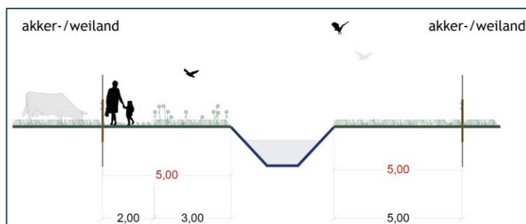
Dwarsprofiel 3
