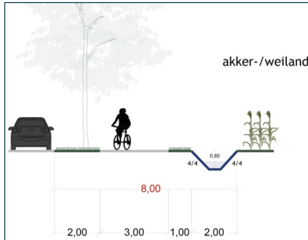
Dwarsprofiel 12 (fietspad 42)
