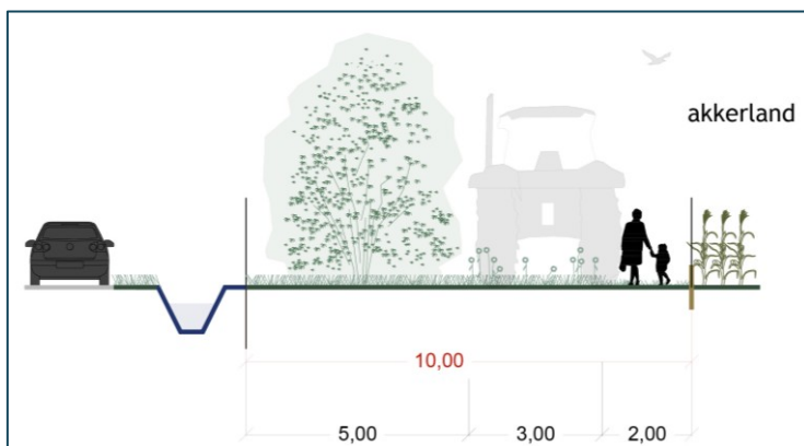
Dwarsprofiel 5
