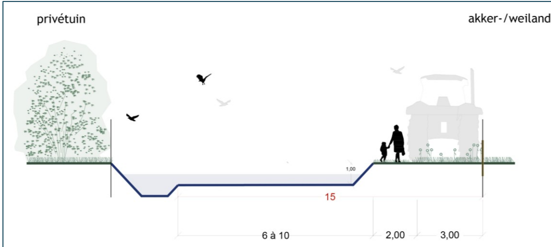
Dwarsprofiel 14
