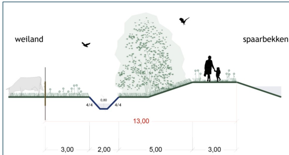
Dwarsprofiel 7
