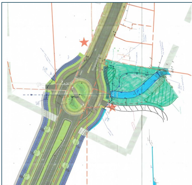
Ontwerpschets toegangspoort Hoogstade, ©Sweco (februari 2026)
