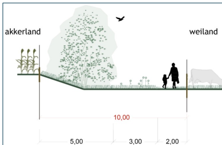
Dwarsprofiel 4
