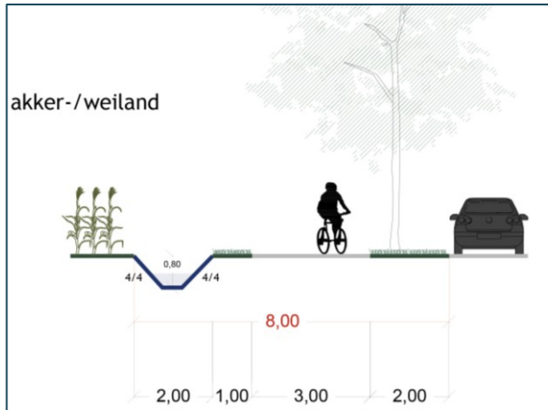
Dwarsprofiel 11 (fietspad 37)
