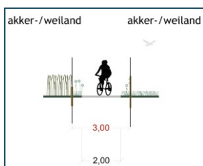
Dwarsprofiel 1
