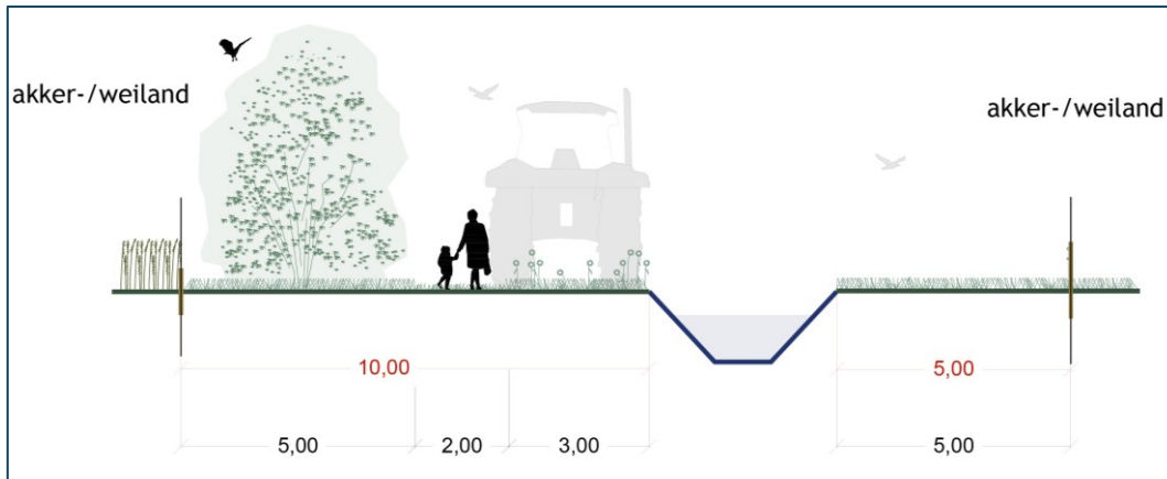
Dwarsprofiel 2
