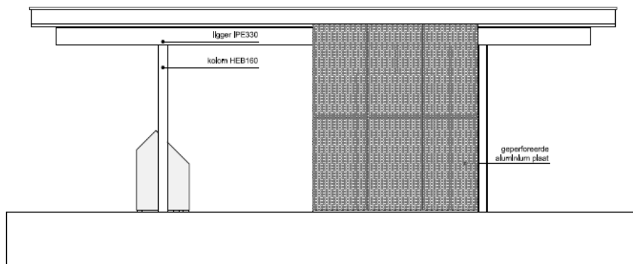
AANZICHT BA
