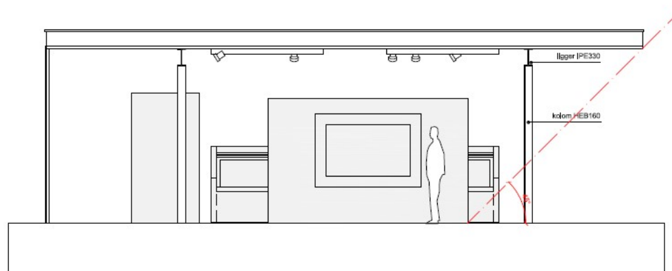
AANZICHT AD
