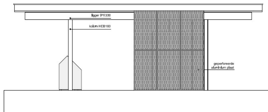
AANZICHT BA
