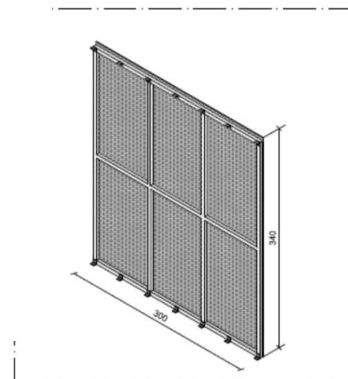
GEPERFOREERDE PLAAT MET DRAAGSTRUCTUUR
