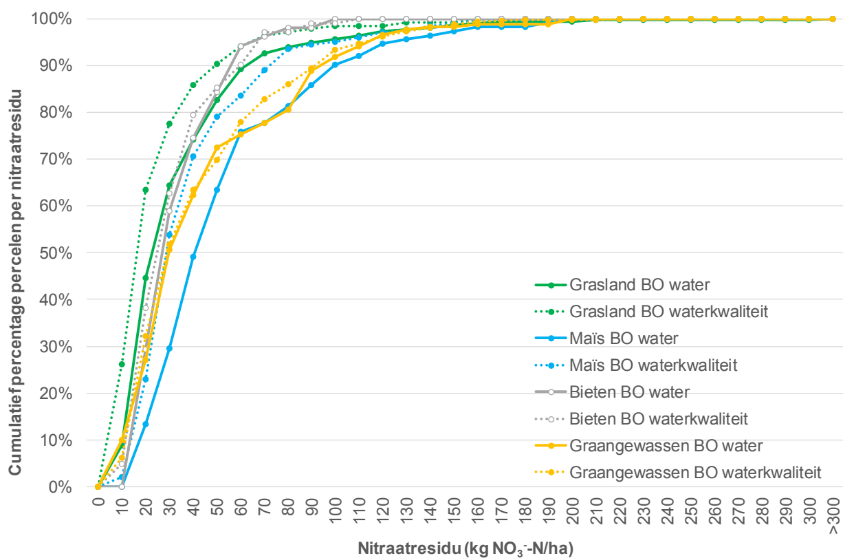
Figuur 42 Cumulatief percentage percelen met een bepaald nitraatresidu per teeltgroep, bij de nitraatresidumetingen voor de BO water en de BO waterkwaliteit in 2016
